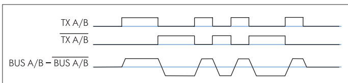
Рис.5. Пример преобразования сигнала передатчиком ИС типа HI-1567
