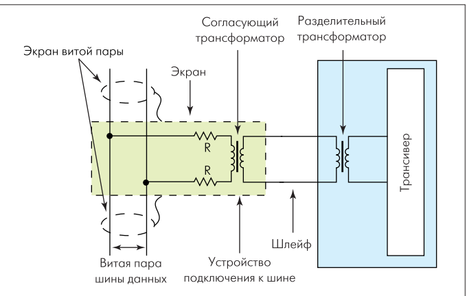
Рис.6. Схема подключения устройства к шине данных посредством согласующего трансформатора
