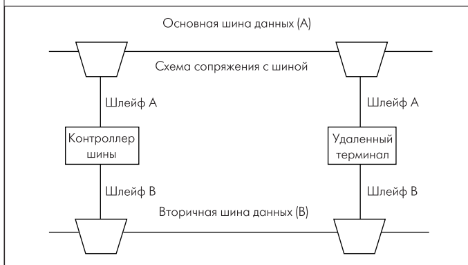
Рис.3. Применение двух шин в сети стандарта MIL-STD-1553
